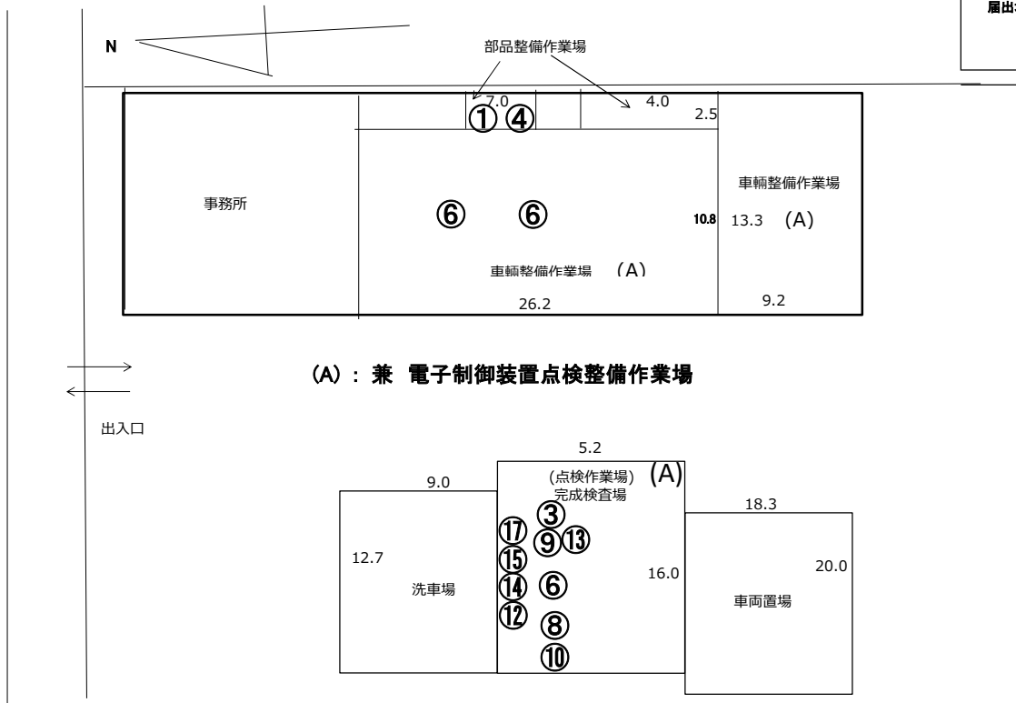
②自動車検査用機械器具の配置状況 (1/100) 単位：m
