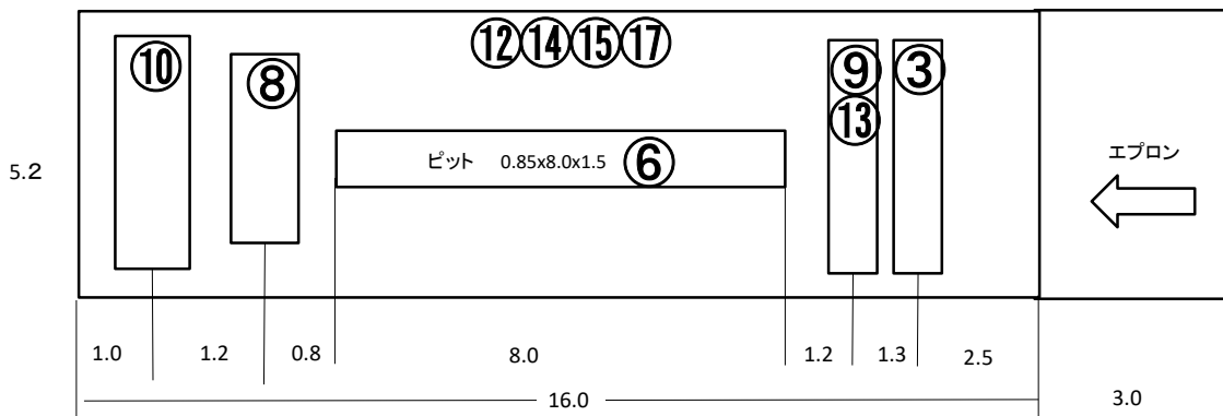
②自動車検査用機械器具の配置状況 (1/100) 単位：m
