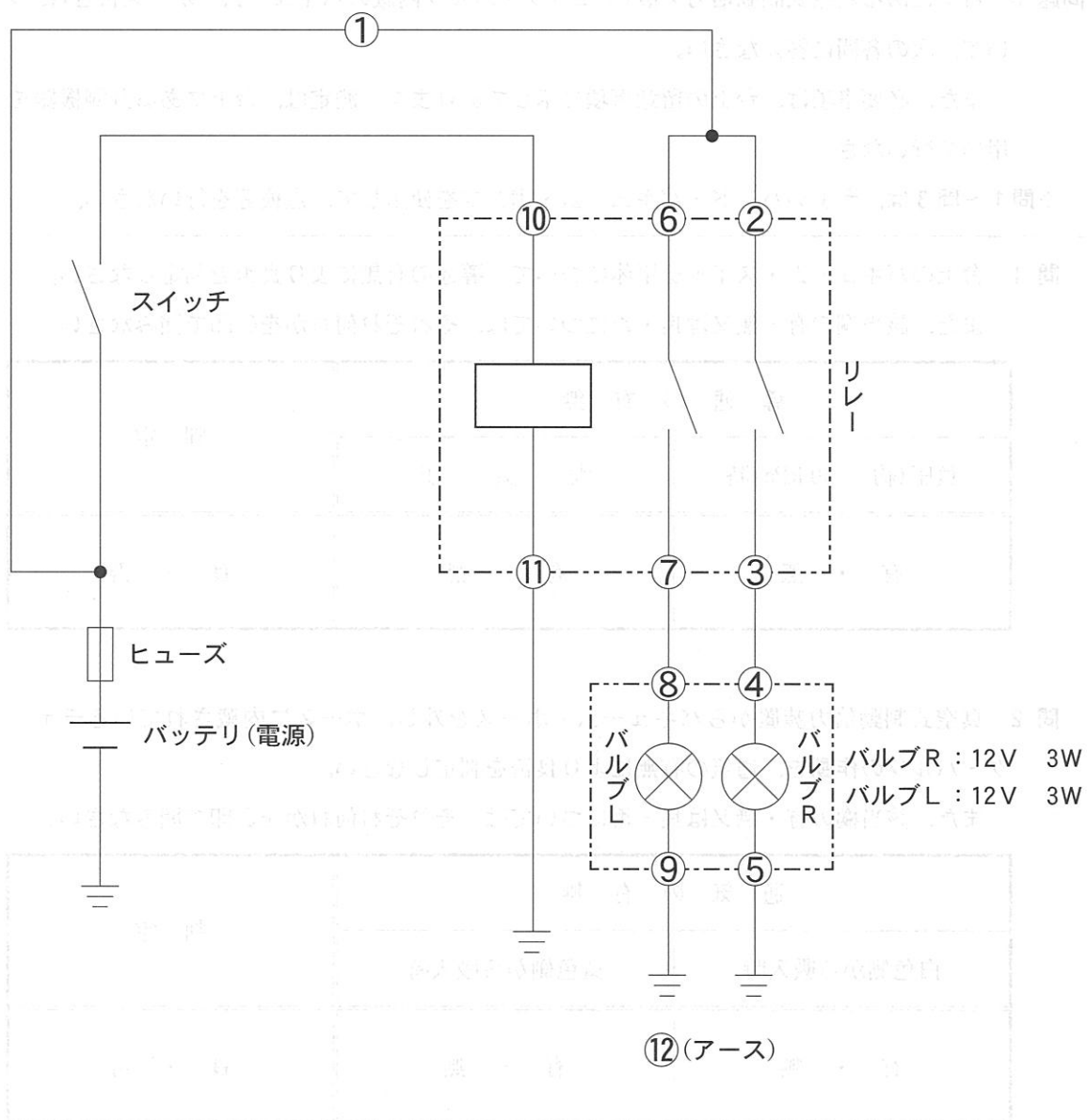
〈リレー回路の回路図〉
